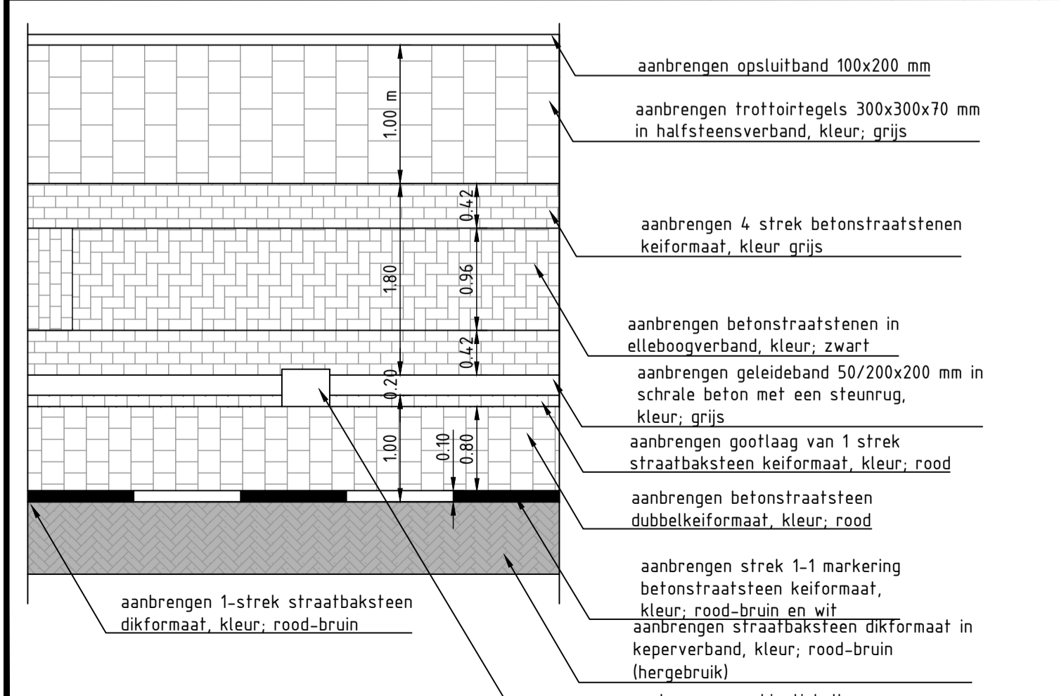
Principedetail langspaarkeerstrook SCHAAL 1 : 50
